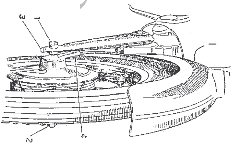
Fig. 12. - Fissaggio ruota anteriore:
