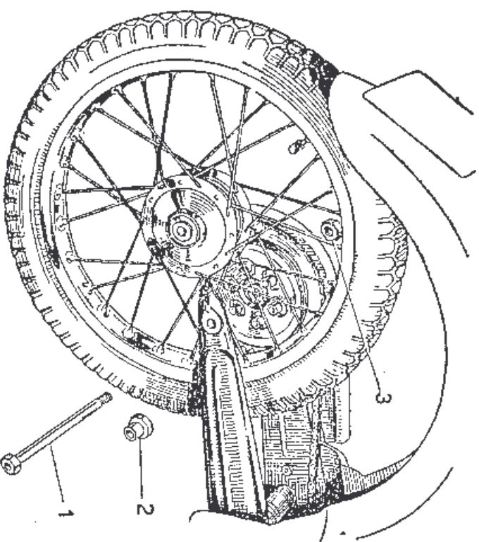
Fig. 14. - Smontaggio ruota posteriore.
