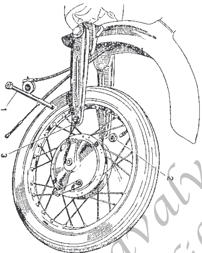
Fig. 13. - Smontaggio ruota anteriore.
