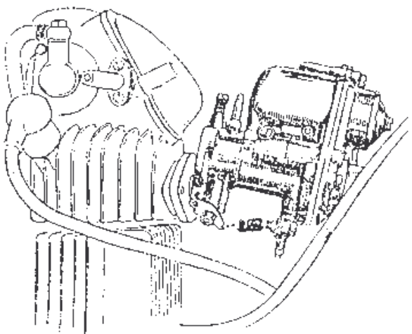
Fig. 18. - Rimozione del carburatore dal motore.
