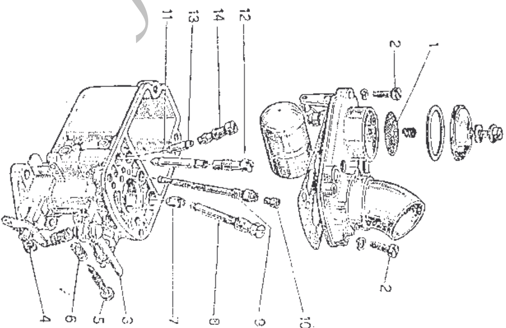
Fig. 19. - Carburatore Weber 22 DZM smontato per la pulizia
