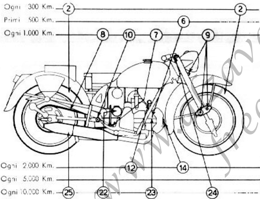
SCHEMA DELLA MANUTENZIONE (I numeri si riferiscono alle operazioni della « Tabella riassuntiva della manutenzione »)
