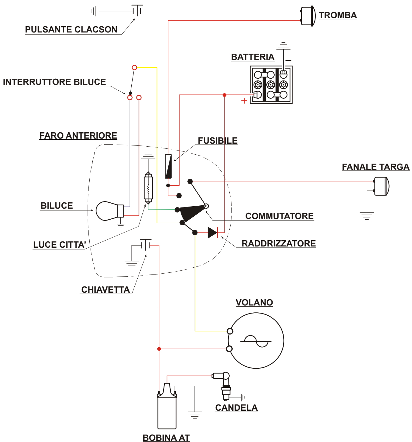
SCHEMA IMPIANTO ELETTRICO CECCATO 125 4T
